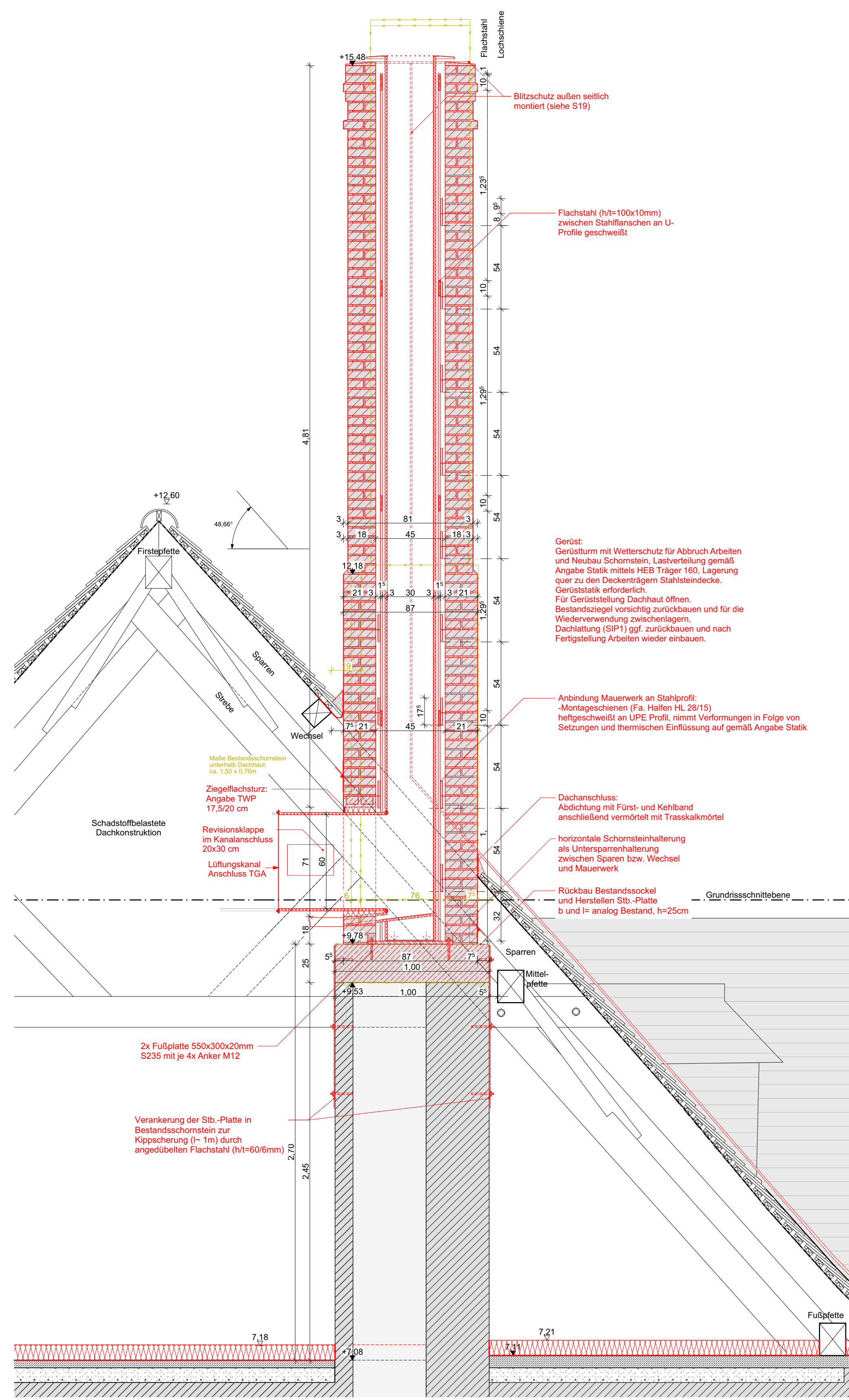
Schnitt A-A 1:20
