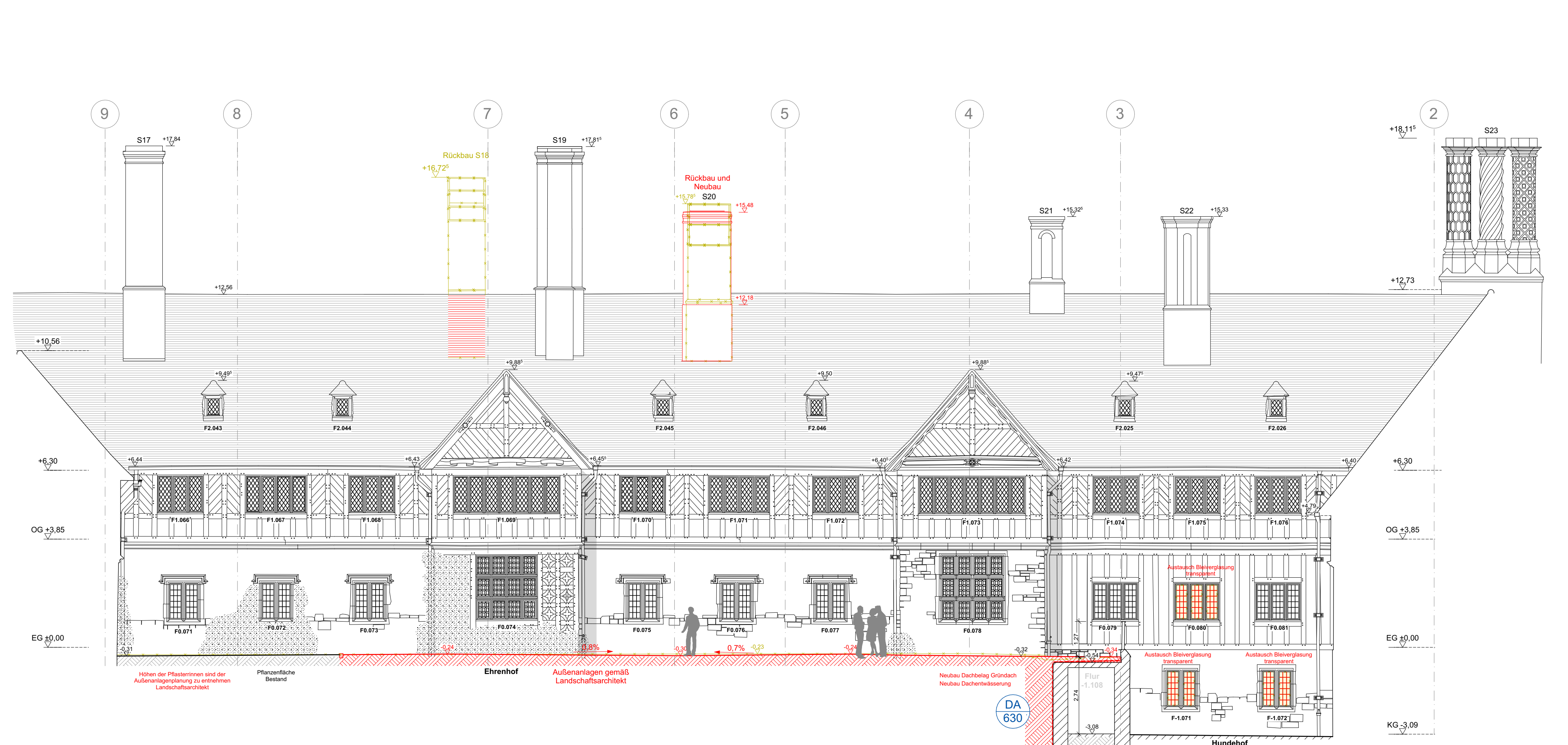
Ehrenhof Westflügel Ansicht Ost 1:100
