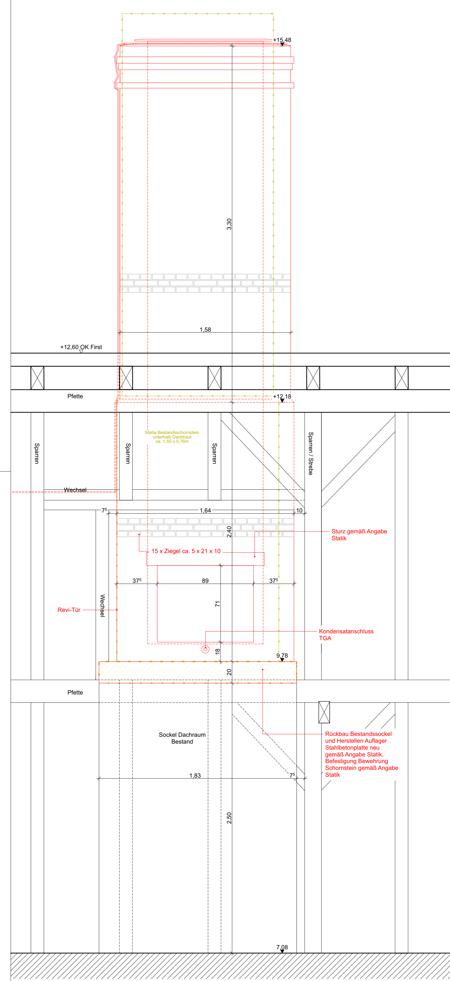
Ansicht West 1:20
