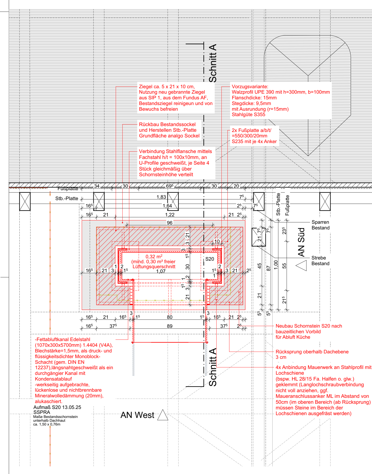
Grundriss 1:20
