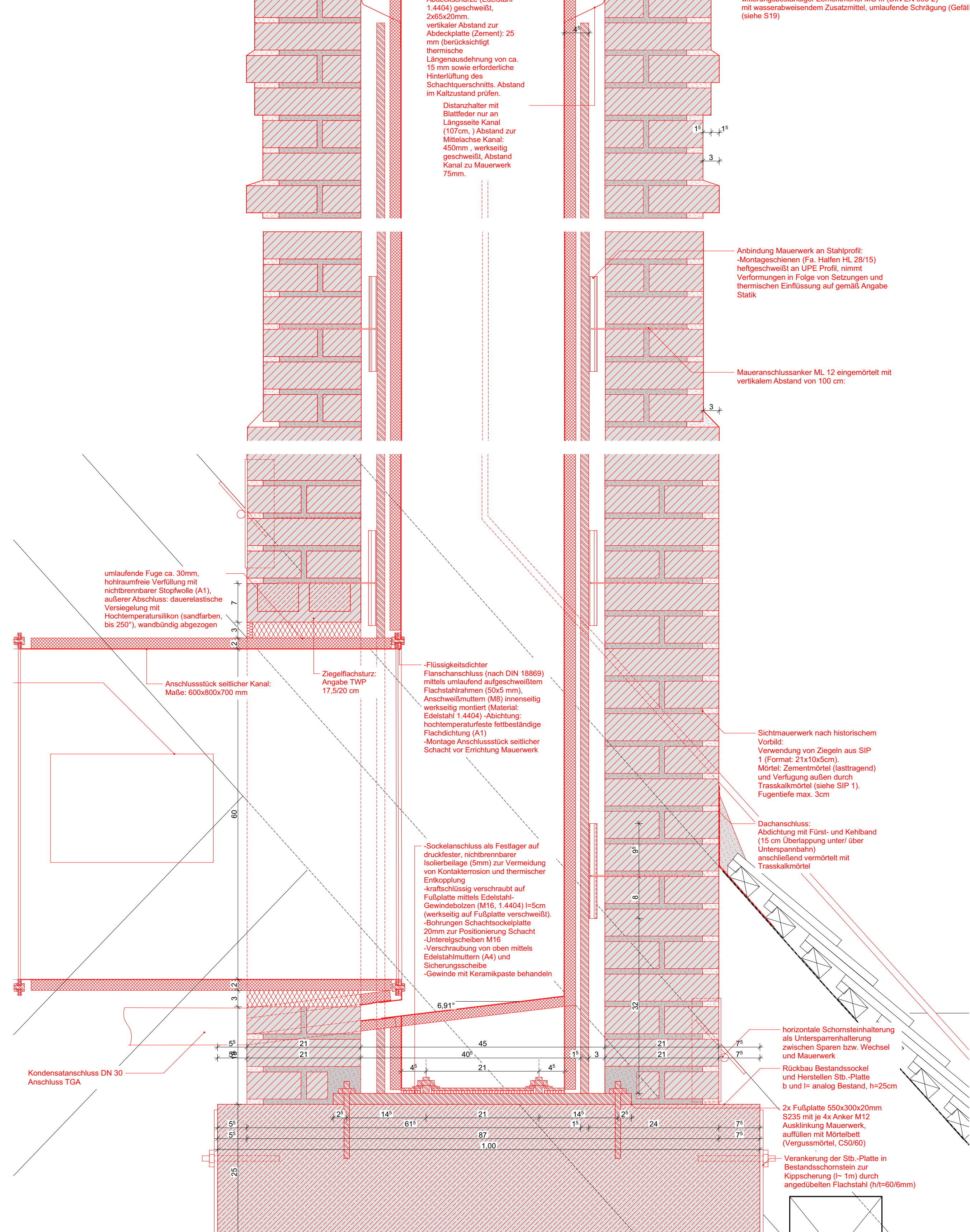
Detail Schnitt A-A 1:5
