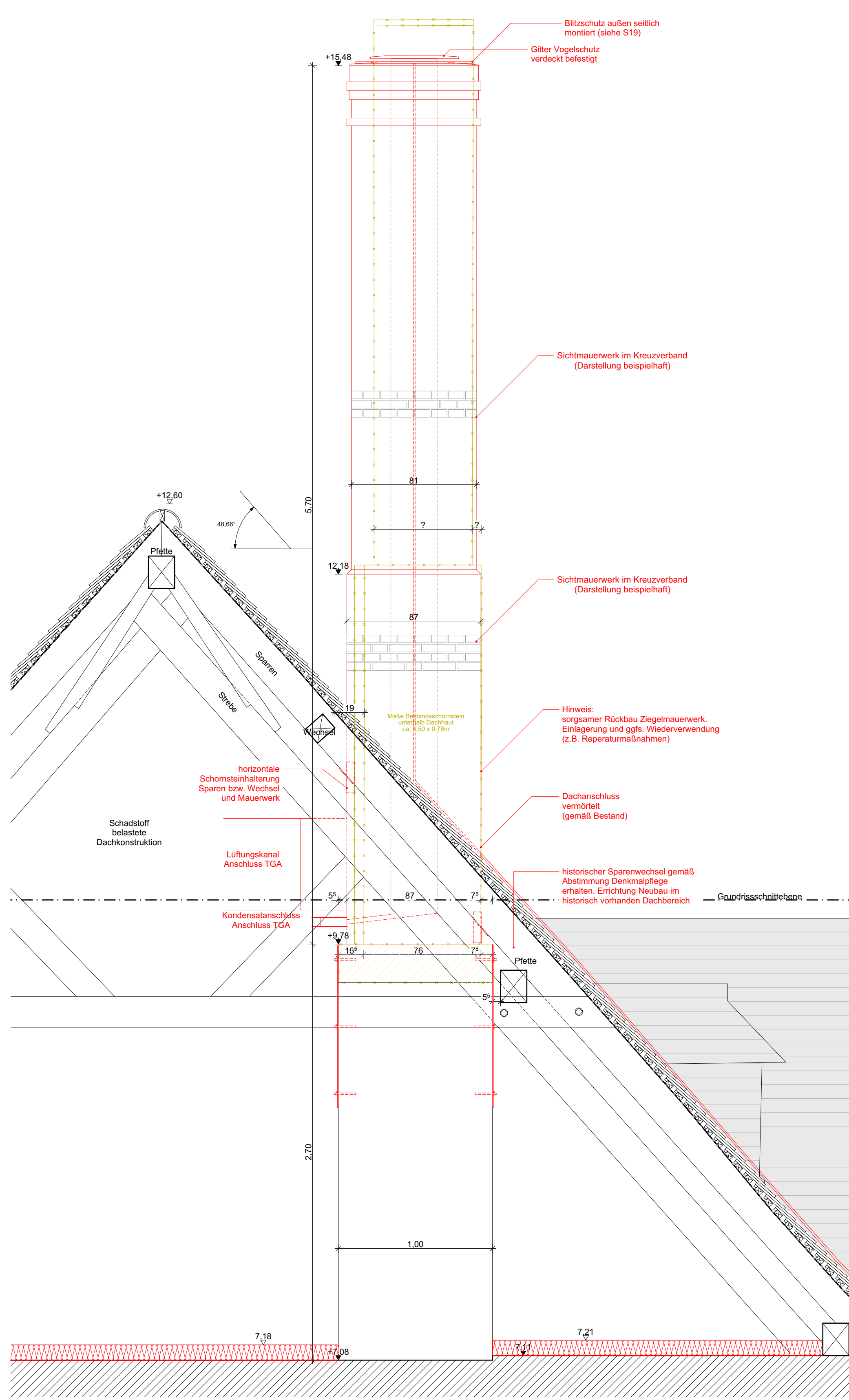
Ansicht Süd 1:20
